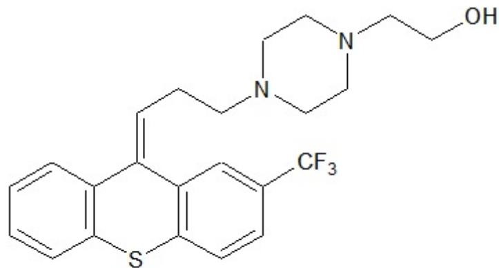
cis-form
